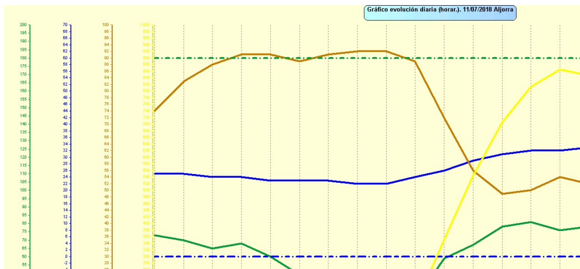
Gráfica 8.- Evolución diaria-horaria del día 11/07/2018 en la estación de inmisión de Aljorra para el contaminante ozono y el resto de los parámetros meteorológicos. Tipo: Suburbana
