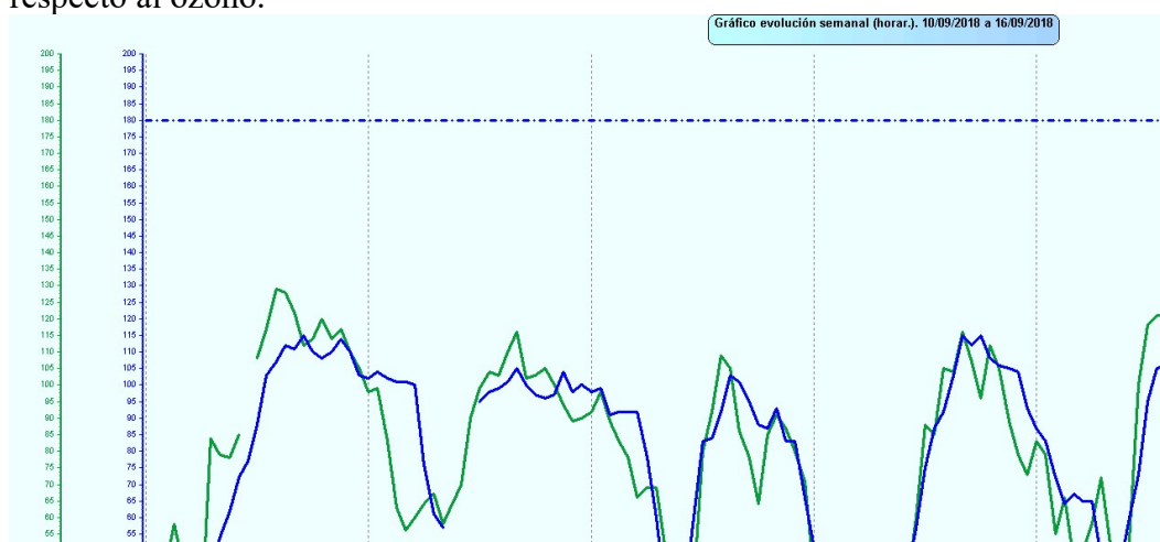
Gráfica 5.- Evolución semanal horaria desde el día 10/09/2018 hasta el día 16/09/2018 en las estaciones de inmisión de La Aljorra y Alumbres para el contaminante ozono. Tipo: Suburbana
